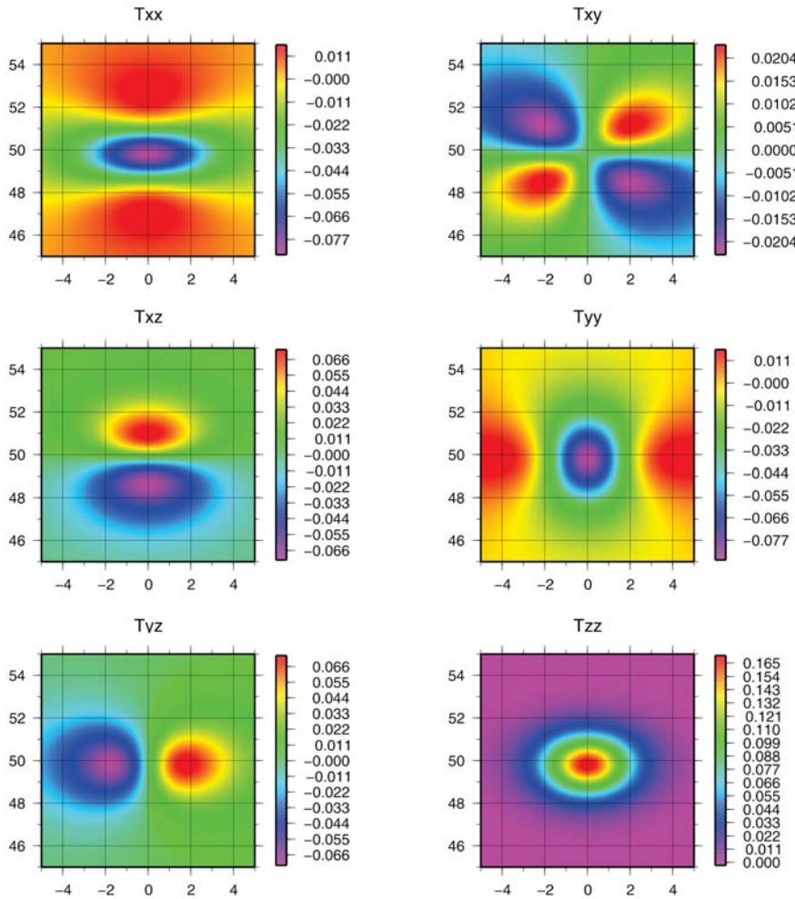
Figura 5: TGG generado utilizando un tesoroides de 1° x 1° x 1 km, n_x = m_\varphi = p_r = 8 , y una altura de cálculo de 250 km; calculado con el programa Tesseroids (Uieda et al. 2010), el cual utiliza prismas esféricos para el cálculo. La escala está en Eötvös.
