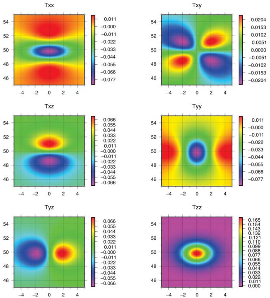
Figura 4: TGG generado utilizando una topografía sintética de 1° x 1° x 1 km, n_s = m_p = p_r = 8 , y una altura de cálculo de 250 km; calculado con el programa Tesseroide-V2 luego de transformar la topografía sintética en teseroides con el programa DEM2tess , el cual utiliza prismas esféricos para el cálculo. La escala está en Eötvös.
