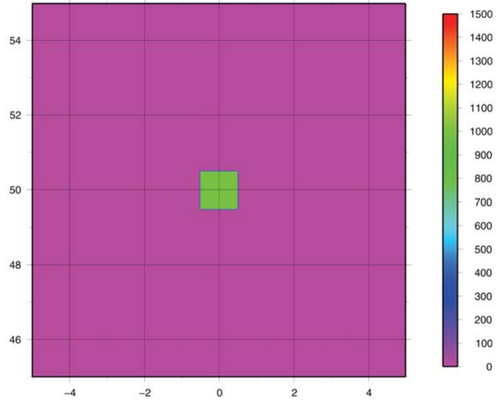
Figura 3: Prisma de 1° x 1° con 1 km de altura centrado en la latitud de 50°N y longitud 0, que simula una topografía sintética.
