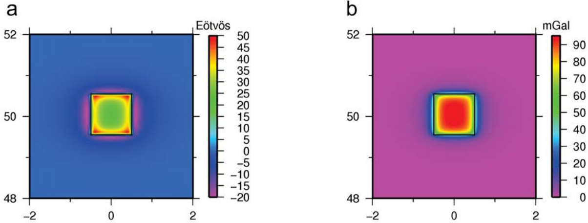
Figura 1: Comparación entre el gradiente vertical de gravedad ( T_{zz} ) y la anomalía gravimétrica ( Ga ) para un prisma. El cuadrado centrado en 0^\circ \pm 0.5^\circ y en 50^\circ \pm 0.5^\circ representa la posición del prisma para el cual son calculados ambos efectos. a) Gradiente vertical de gravedad. b) Anomalía de gravedad.
